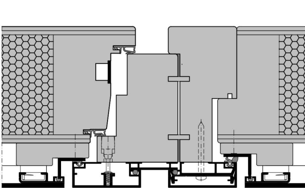
Pfosten mit Lüftungsklappe und Paneelfeld
